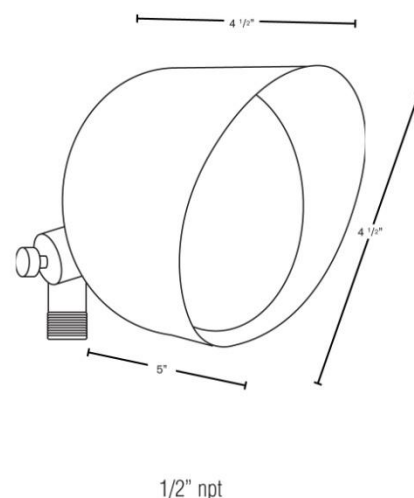
FL-117B-PAR36
